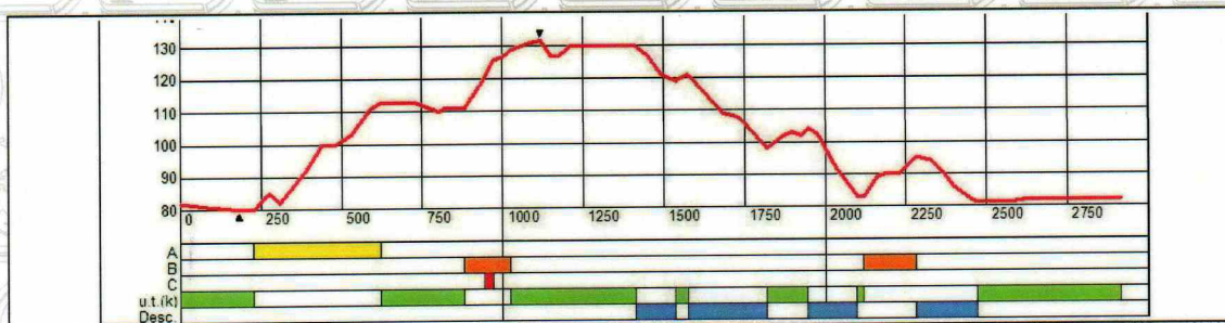
Профиль трассы
